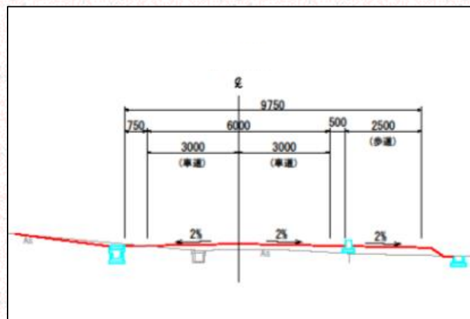
標準断面図
