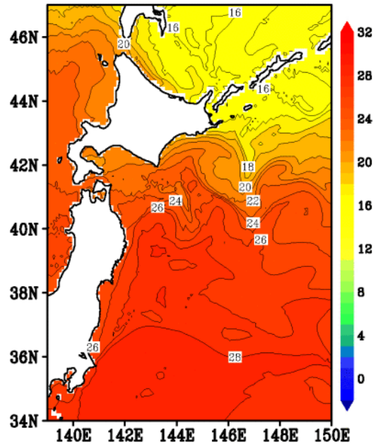
b) 北海道・東北ブロック(139-150E,34-47N)/2025年08月03日/水温/0m
