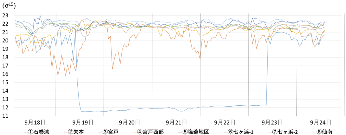
自動観測ブイによる 比重 の推移
