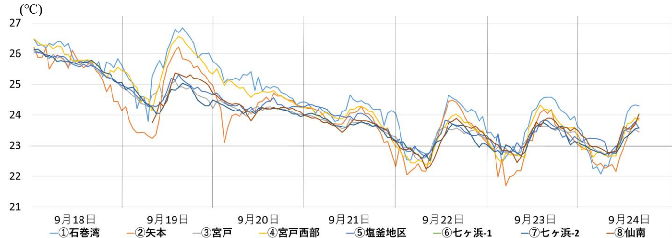
自動観測ブイによる 水温 の推移
